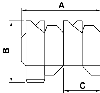
Faltboden
